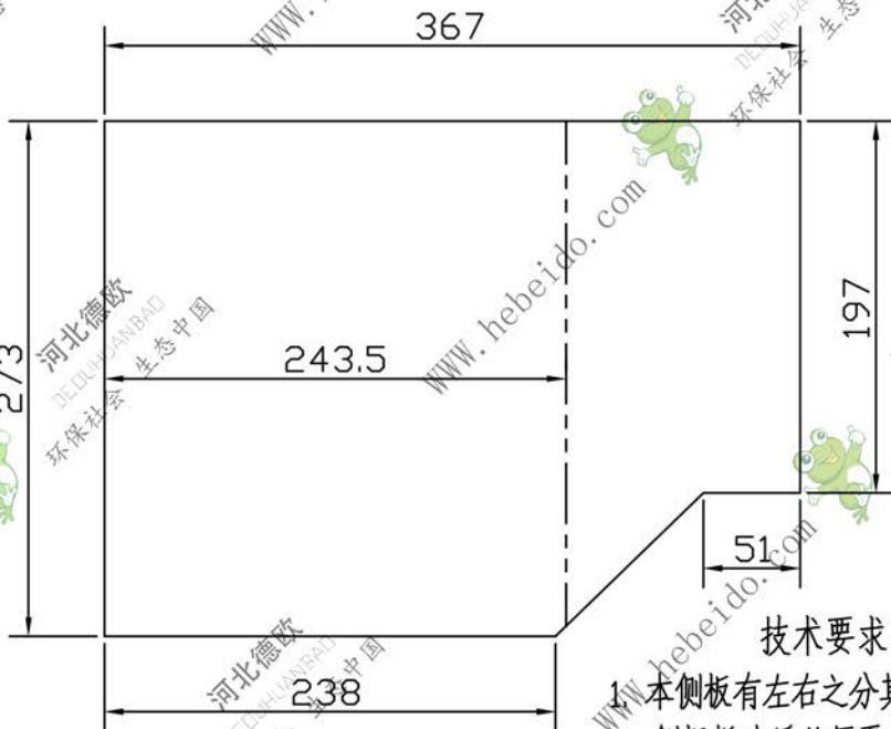
展开图
