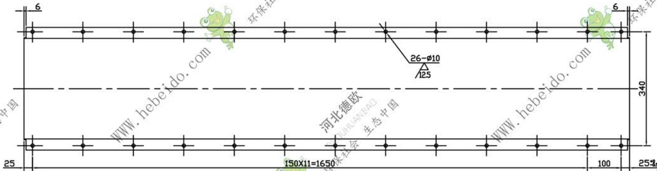
展开图
