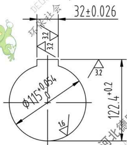
轴孔图
